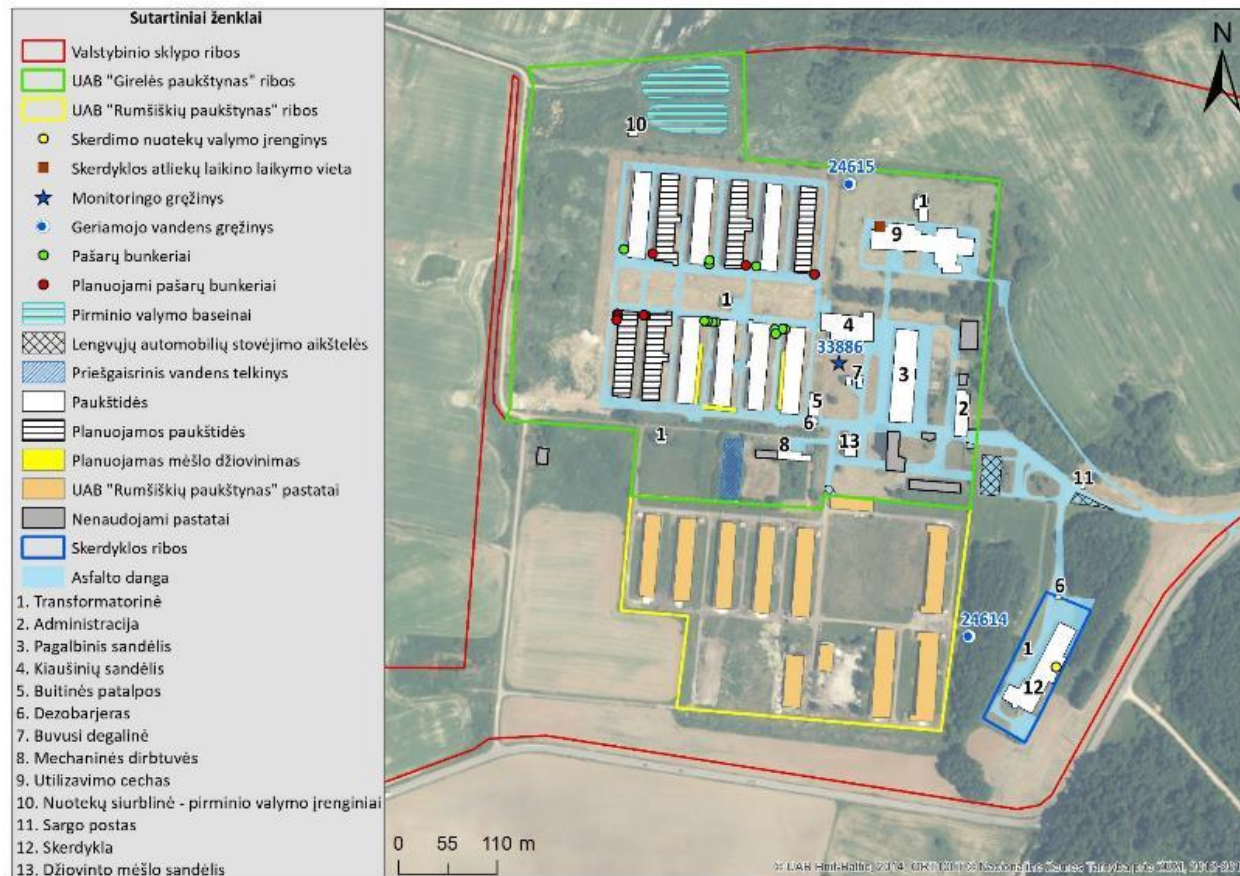
10 pav. UAB „Girelės paukštynas“ gamybinės teritorijos bei esamų ir planuojamų technologinių statinių ir įrenginių išdėstymo planas
